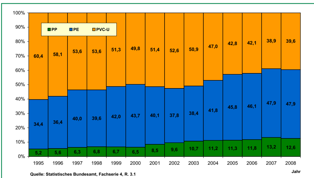
Abbildung 3: Marktanteile der Kunststoffrohrwerkstoffe PP, PE und PVC-U in % der Gesamt- kunststoffrohrpro- duktion Deutschland
