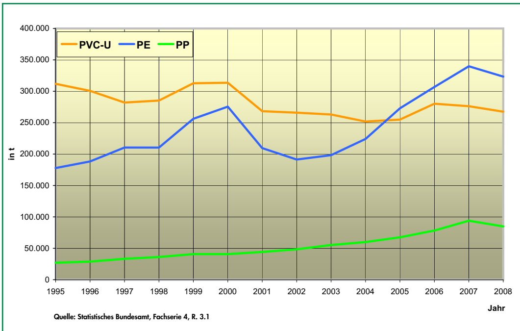
Abbildung 2: Produktion von PE-, PVC-U- und PP-Rohren
