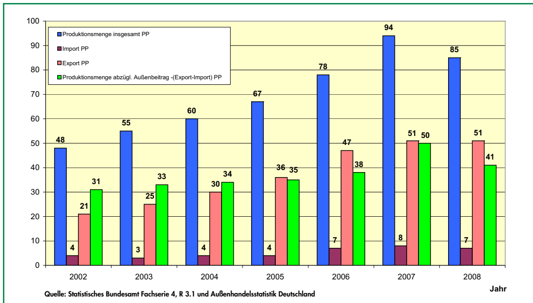
Abbildung 7: Produktion Kunststoffrohrsysteme aus PP nach Verwendung Gesamt, Inland, Export, Import in 1.000 t
