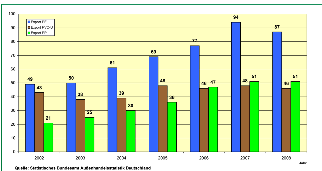
Abbildung 6: Export Rohrleitungssysteme aus PE, PVC-U, PP der Produktionsmenge in 1.000 t
